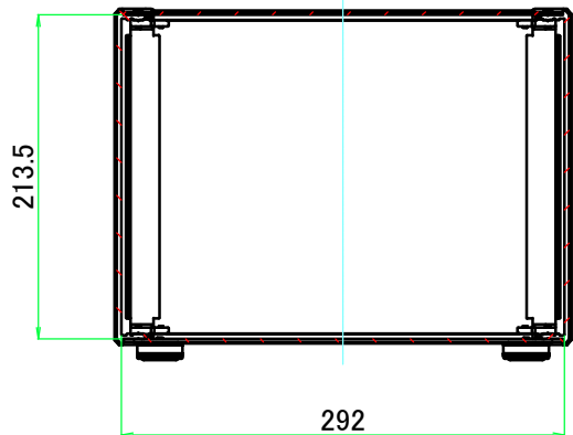
A-A ( 1 : 5.5 )
